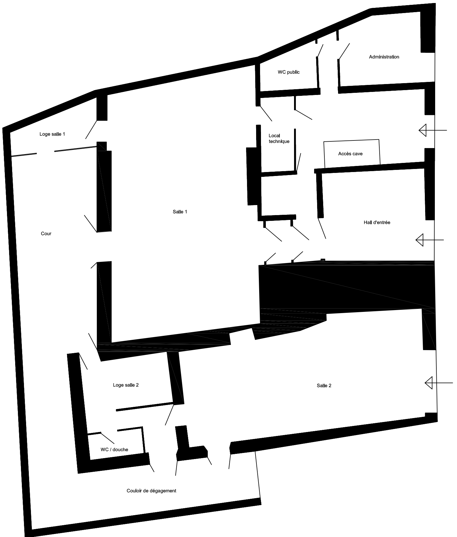
Théâtre Transversal Vue générale de dessus Echelle : 1/100°
